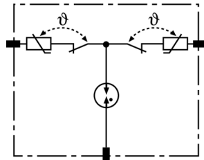
Prinzipschaltbild DR MOD 30
