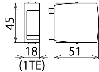
Maßbild DR MOD 30
