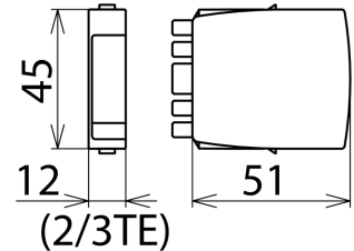
Maßbild BXT ML4 BC EX 24
