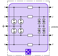
Principalschaltbild BXT ML4 BC EX 24
