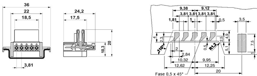
Detailmaßbild der Tragschienen-Busverbinder-Kontaktpads
