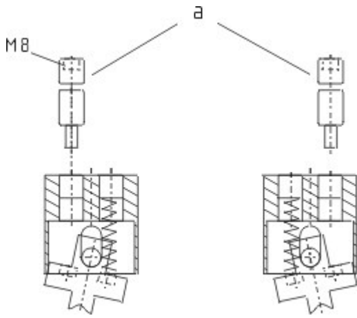
Maßzeichnung (Sonstige)
