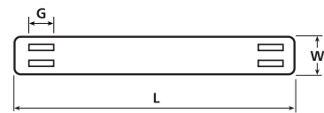
Kennzeichnungsschild AT2
