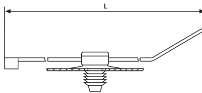
Befestigungsbinder mit Lamellenfuß
