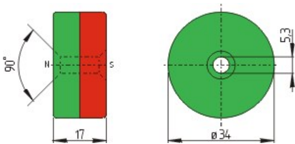
Maßzeichnung (Sonstige)
