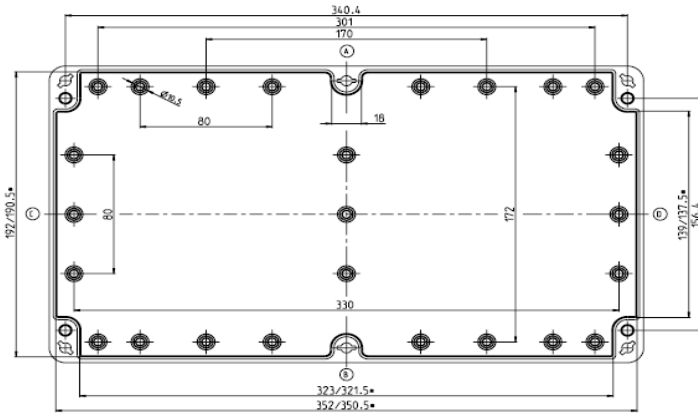
Unterteil
