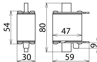
Maßbild VA NH00 280
