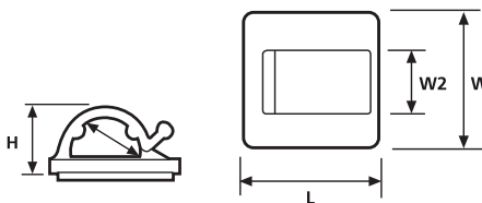
Befestigungssockel RB5-14
