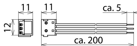
Maßbild BT 24
