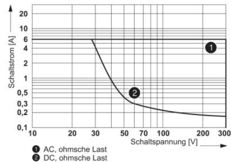
Abschaltleistung
