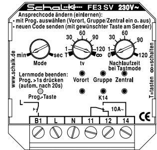
FE3 S(V) Empfänger mit 1 Relais
