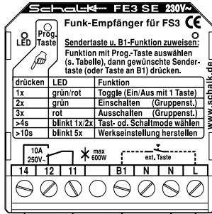
FE3 SE Empfänger mit 1 Relais
