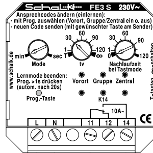
FE3 S(V) Empfänger mit 1 Relais
