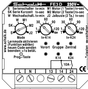
FE3 D(V) Empfänger mit 2 Relais
