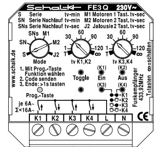
FE3 Q Empfänger mit 4 Relais
