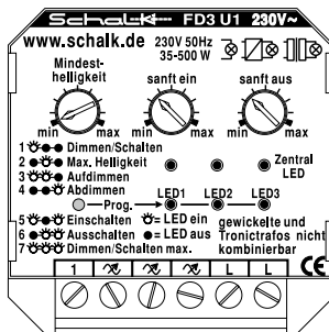
FD3 U1 Universaldimmer
