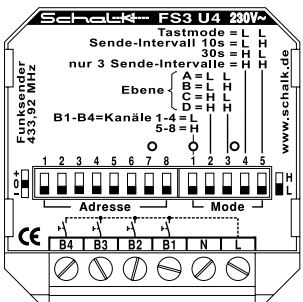
FS3 U4 Einbausender
