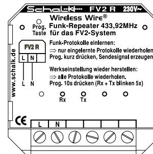
Repeater optional
