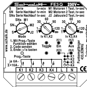
FE3 Q Empfänger mit 4 Relais
