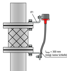
Einbauvariante EXFS L100
