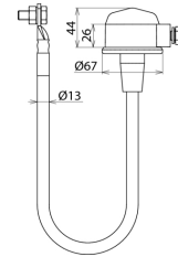
Maßbild EXFS L200
