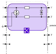
Prinzipschaltbild BXT ML2 BD 180
