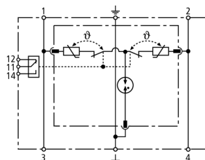
Prinzipialschaltbild DR M 2P 150 FM
