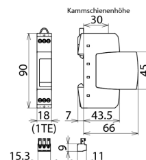
Maßbild DR M 2P 150 FM
