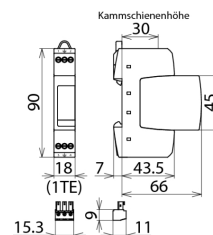
Maßbild DR M 2P 30 FM
