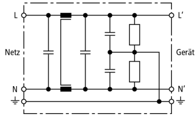
Prinzipschaltbild NF 10
