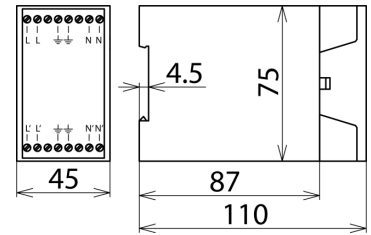
Maßbild NF 10
