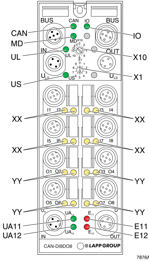
Bild 7 Anzeigen und Drehcodierschalter des Gerätes AB-CAN-DI8DO8-M12-0,5A
