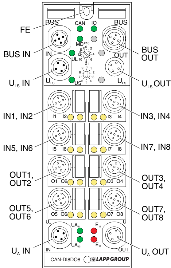
Bild 2 Anschlüsse des Gerätes AB-CAN-DI8DO8-M12-0,5A
