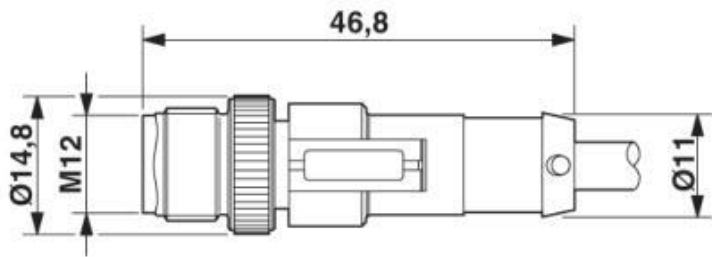
Maßzeichnung Gerader Stecker M12
