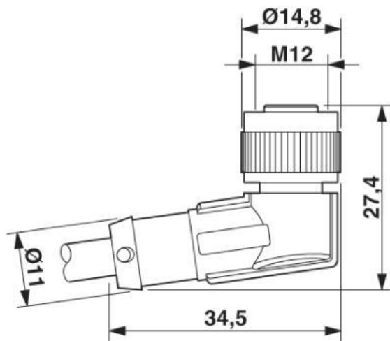
Maßzeichnung gewinkelte Buchse M12
